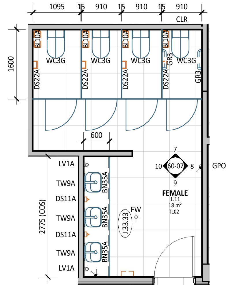
6 PLAN DETAIL 1 : 50
